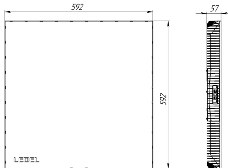
Рисунок 1 Светильник «L-office 32, L-office 55»
